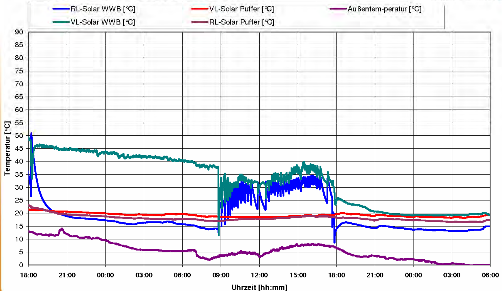
Messung Heizanlage Herbert Kaden 30.03. bis 01.04.2010
