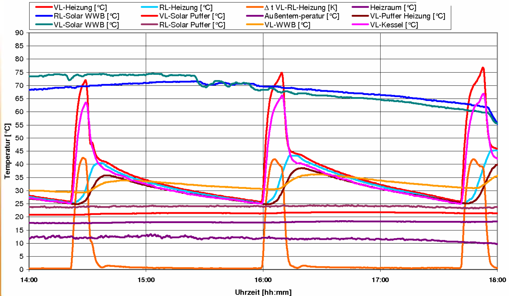
Messung Heizanlage Herbert Kaden 19.04.2010
