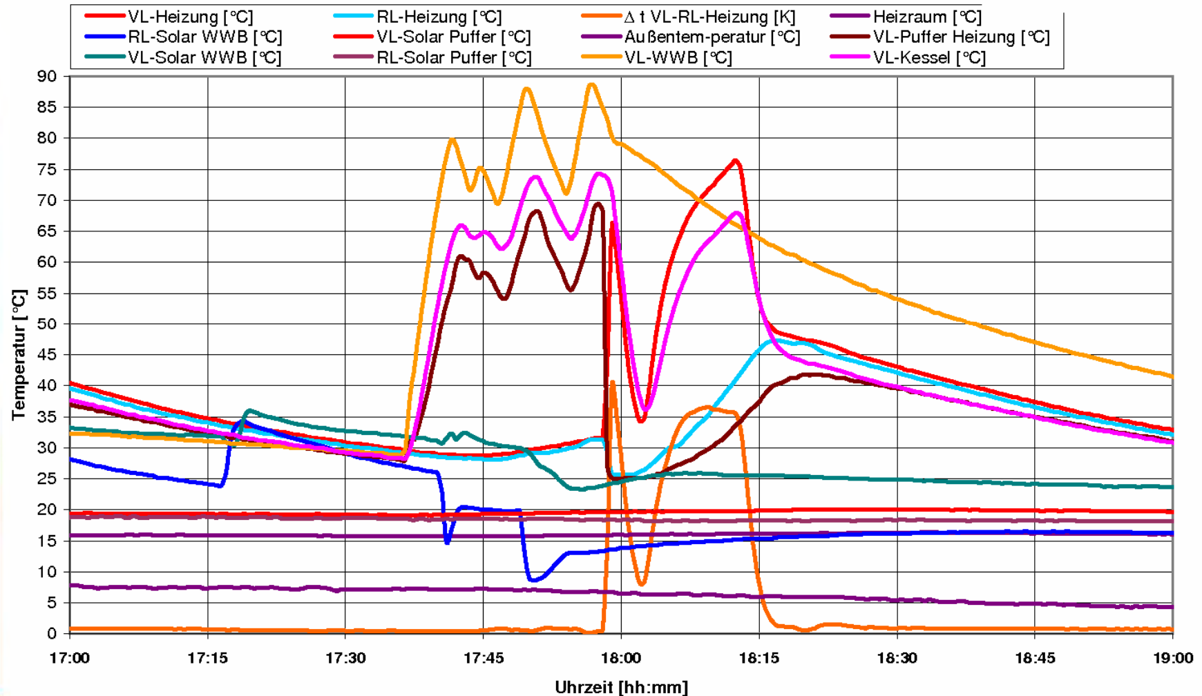
Messung Heizanlage Herbert Kaden 31.03.2010
