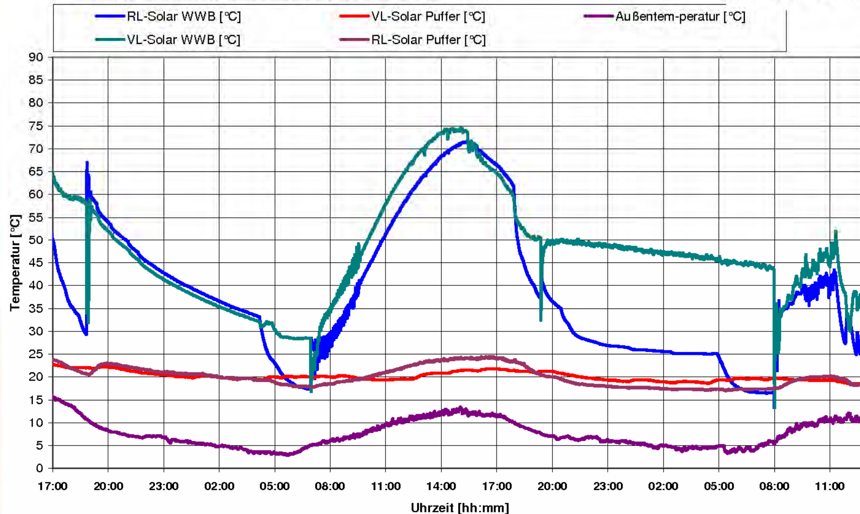
Messung Heizanlage Herbert Kaden 18.-20.04.2010
